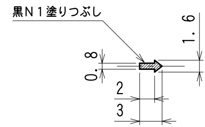
詳細図 2:1
