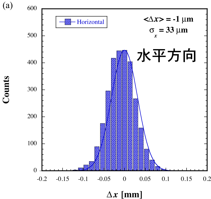
X軸方向の光軸安定度分布
