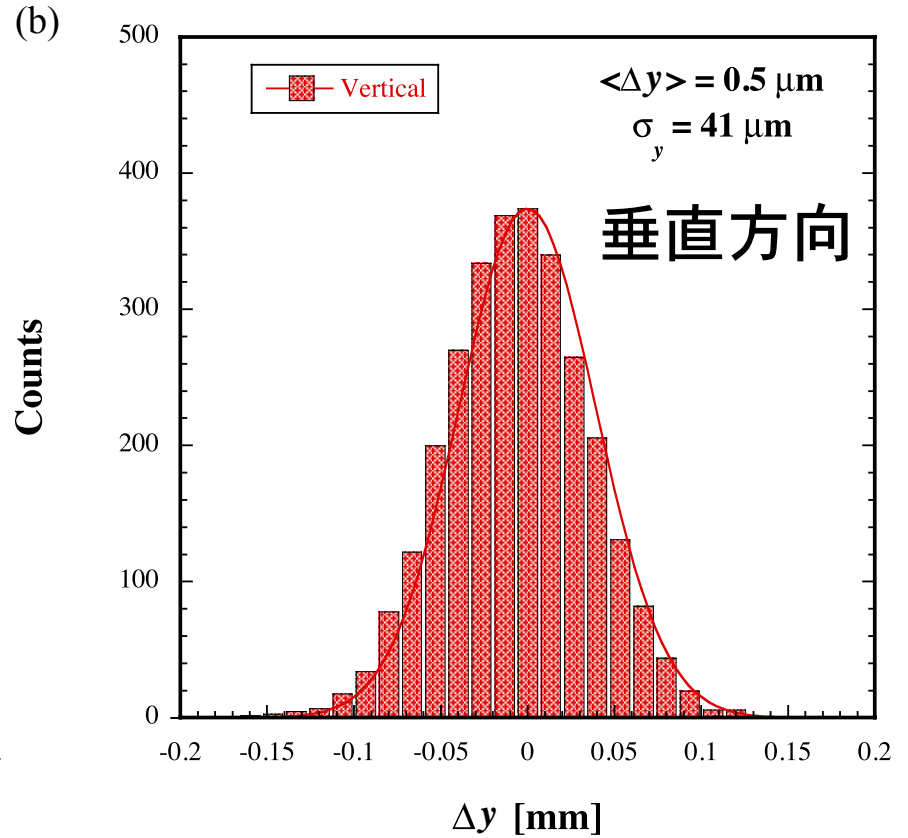
Y軸方向の光軸安定度分布
