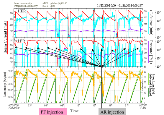
図 4: KEKB 陽電子連続入射時の Daily Snap
