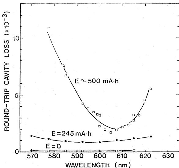
図5 光共振器損失
