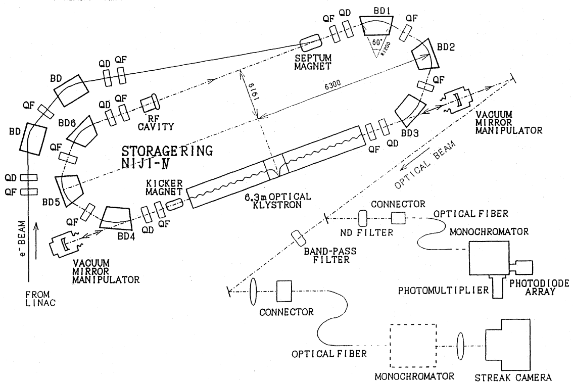
図8 NIJI-IV-FELシステム
