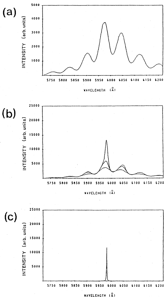
図7 TERAS-FELの出力スペクトル例
