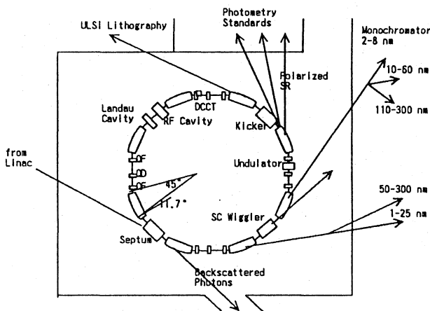
図3 蓄積リング TERAS
