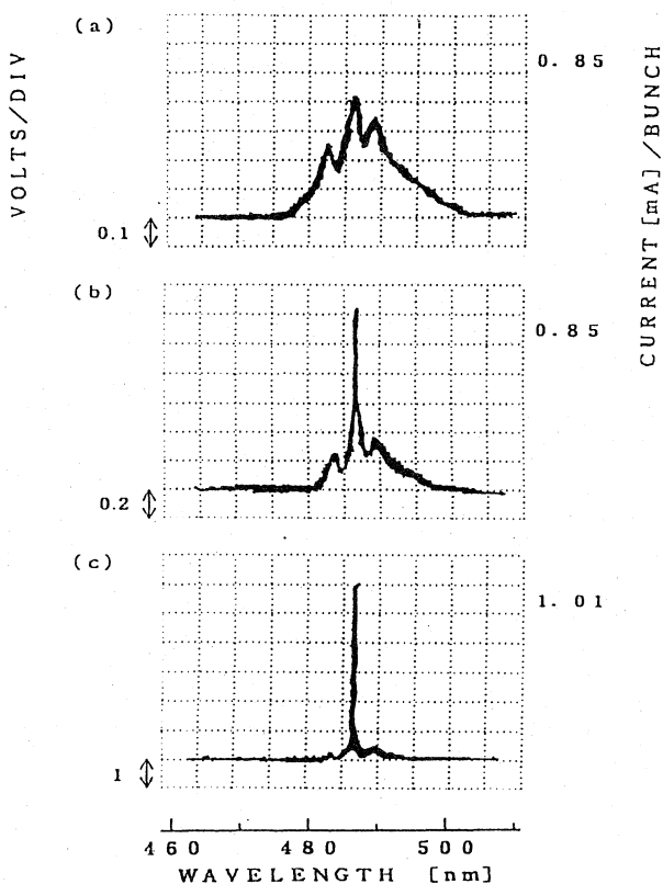
図9 NIJI-IVシステムでの488nmでの発振
