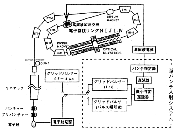
図2 単バンチ入射システム
