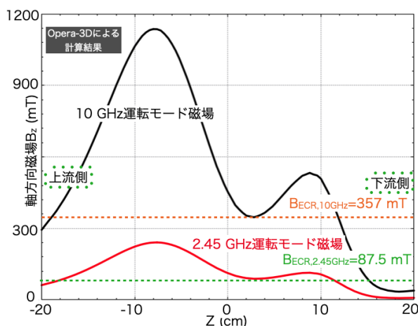
Figure 3: ECR イオン源の設計磁場。
