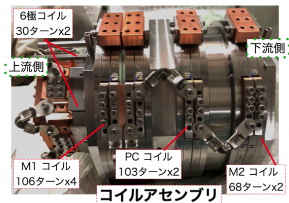
Figure 2: 阪大 RCNP の無絶縁高温超伝導 ECR イオン源のコイルアセンブリ。
