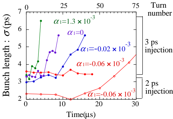
図5 NewSUBARU の \alpha_1 を変えたときの周回毎のバンチ長の変化。
