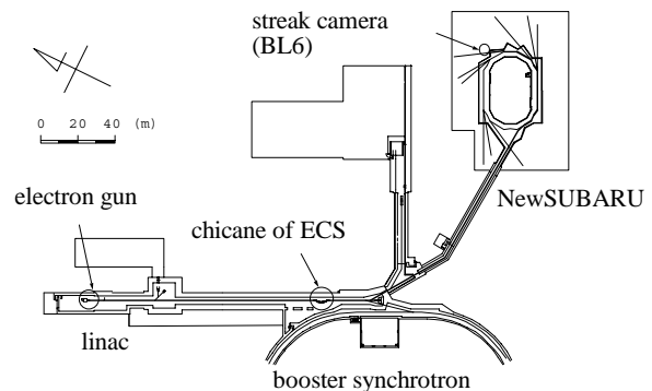
図1 線形加速器とNewSUBARUのレイアウト
