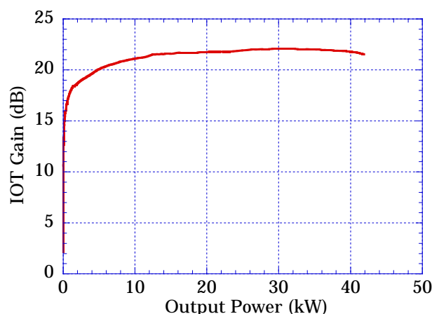
図 1 500MHz-IOT の利得
