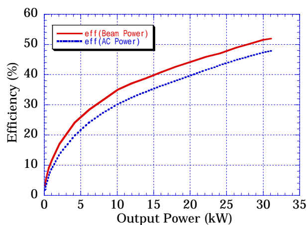
図6 1.3GHz-10Tの効率
