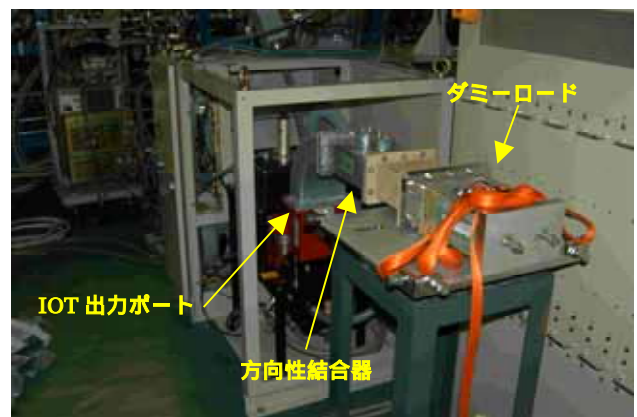
図4 出力試験セットアップ
