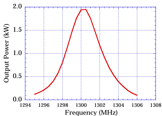
図7 1.3GHz-10Tのバンド幅
