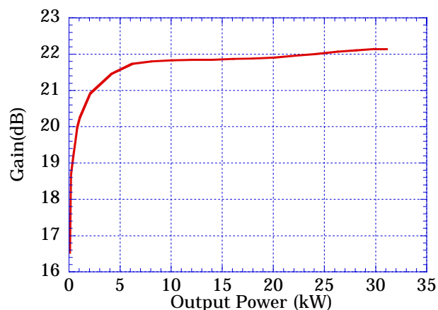
図5 1.3GHz-10Tの利得
