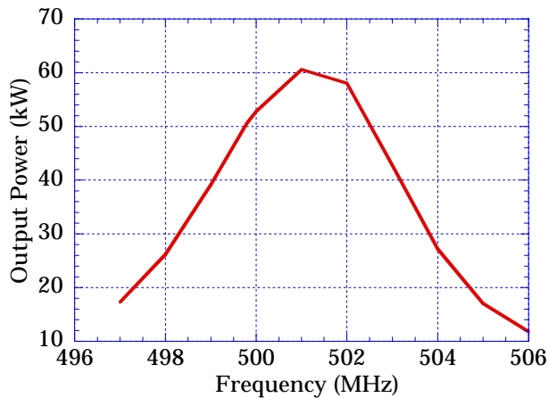
図2 500MHz-10Tのバンド幅
