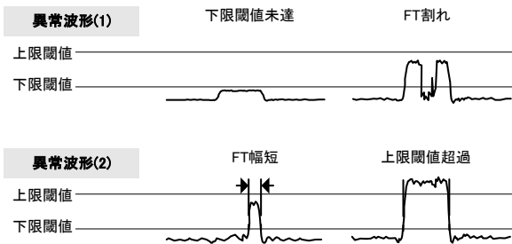
図1 異常波形の種類
