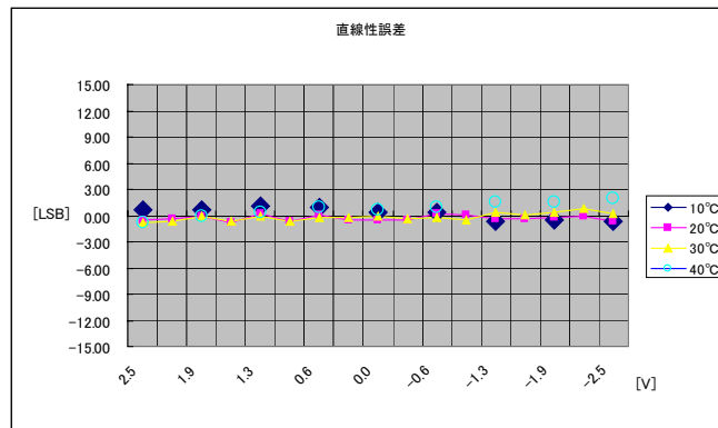
図4. 直線性誤差
