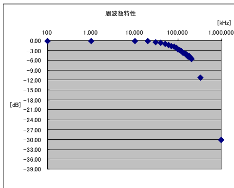
図3. 周波数特性
