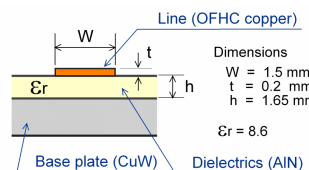
(b) 断面図
