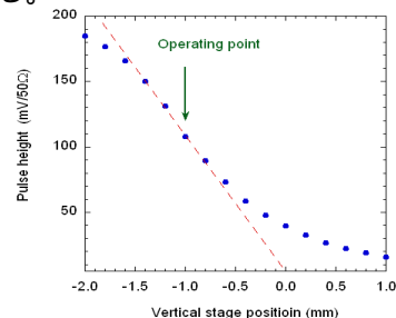
図6：鉛直方向の走査による波高の変化
