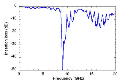
図2：検出素子の高周波特性
