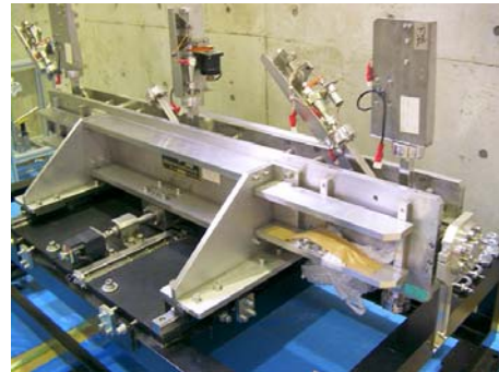
図1 Halbach型アンジュレータ
