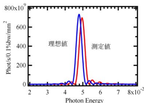
図6 自発放射光スペクトルの基本波部
