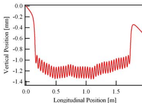
図5 補正をした時のビーム軌道
