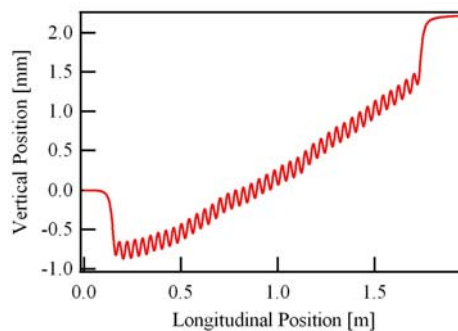
図4 測定値を用いた電子ビーム軌道
