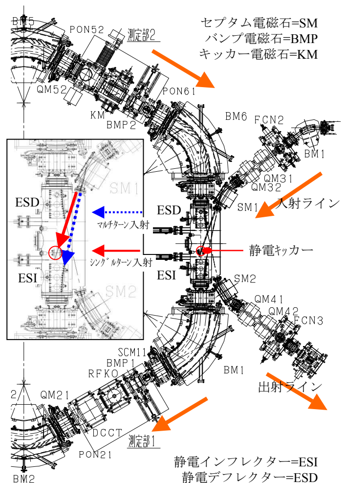
図1: S-LSRの入出射システム
