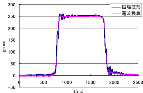
図6: KM磁場パルス波形
