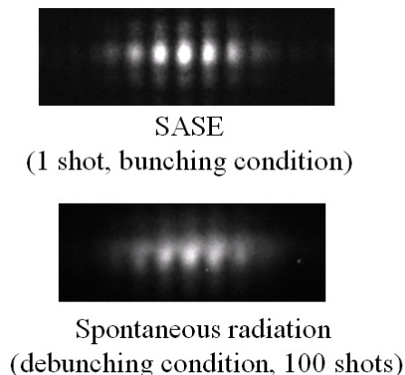
図5. 2重スリットによる干渉試験。 (スリット幅 100 \mu\text{m} , 間隔 400 \mu\text{m} )、SASE増幅では、干渉性の高い波が得られている[12]。
