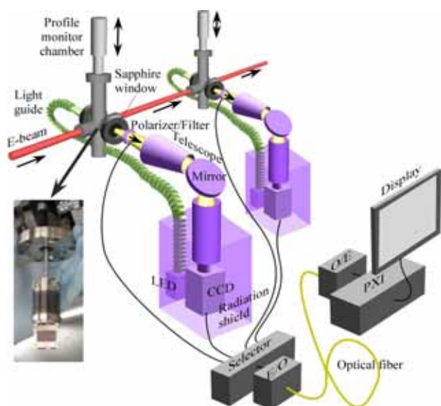
図1. プロファイルモニタシステム構成概略図
