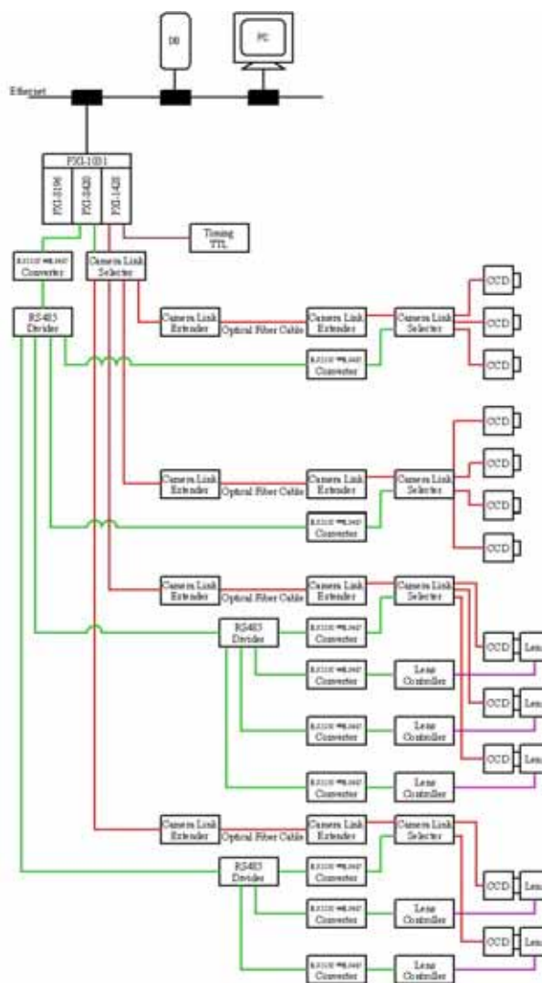
図5 . 配線図
