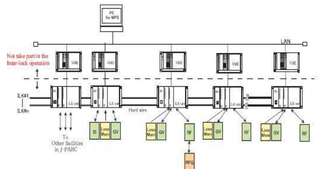
図1. MPSシステム構成例
