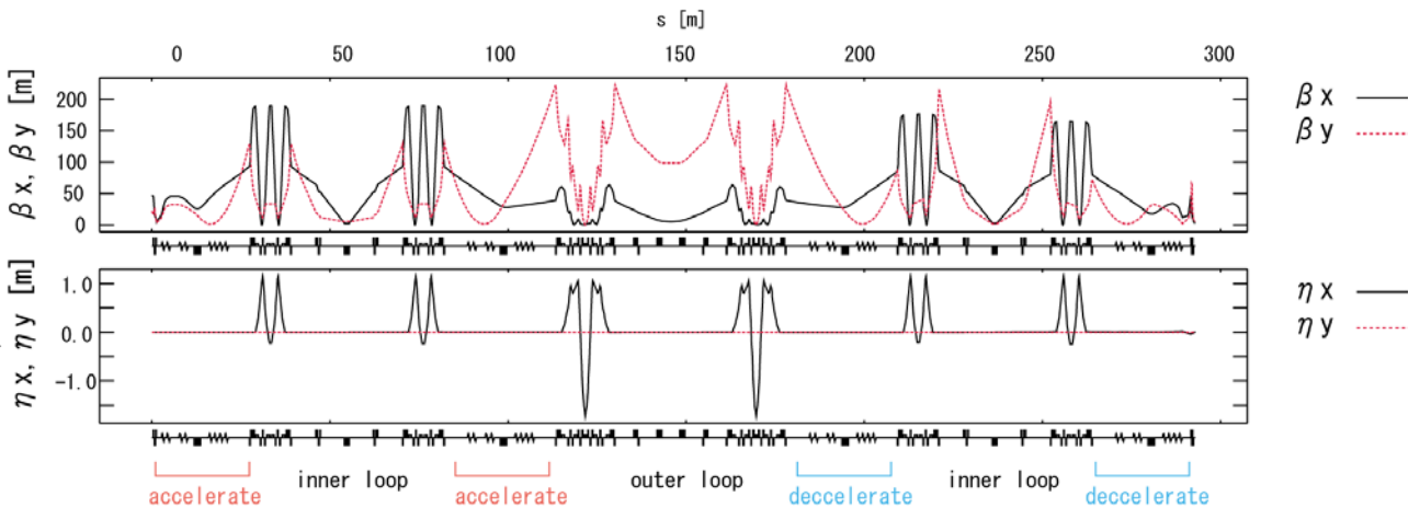
図 5: 入射合流部出口で (\beta_x, \alpha_x, \beta_y, \alpha_y) = (47.1 \text{ m}, 1.65, 21.5 \text{ m}, 5.52) としたときの周回部の線形オプティクス
