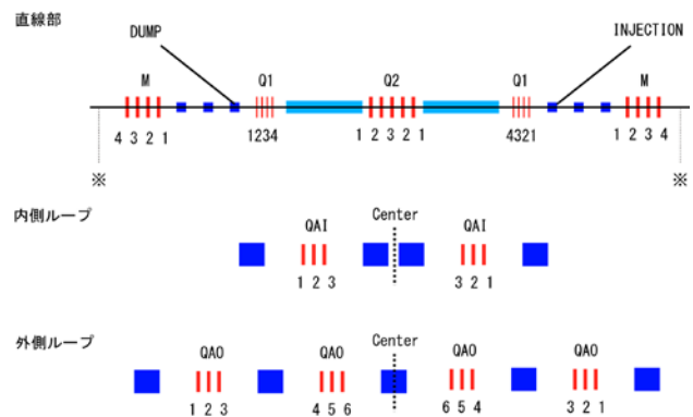
図 3 : 左右対称の光学の設計方針。同じ記号の 4 極電磁石の K 値、および※の twiss parameter は左右対称とする。
