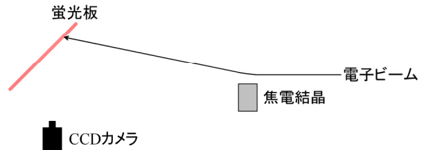
図 6：焦電結晶の電場によるビーム偏向試験の概念図。
