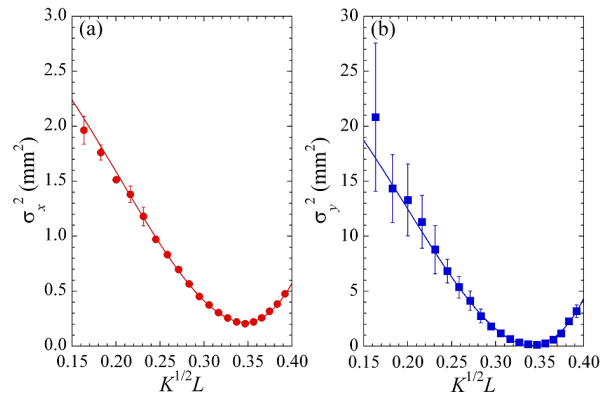
図 7：Q スキャン法の測定結果。横軸： K^{1/2}L ( K は 4 極電磁石の K 値、 L は磁石長)、縦軸：ビームサイズ \sigma の 2 乗。(a) 水平方向、(b) 垂直方向。実線は転送行列から求まる計算式へのフィットを示す。
