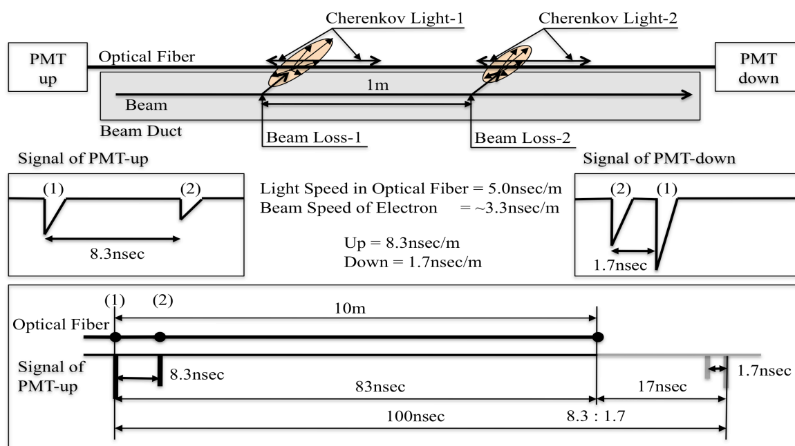
図 1 : 光ファイバー中のチェレンコフ光
